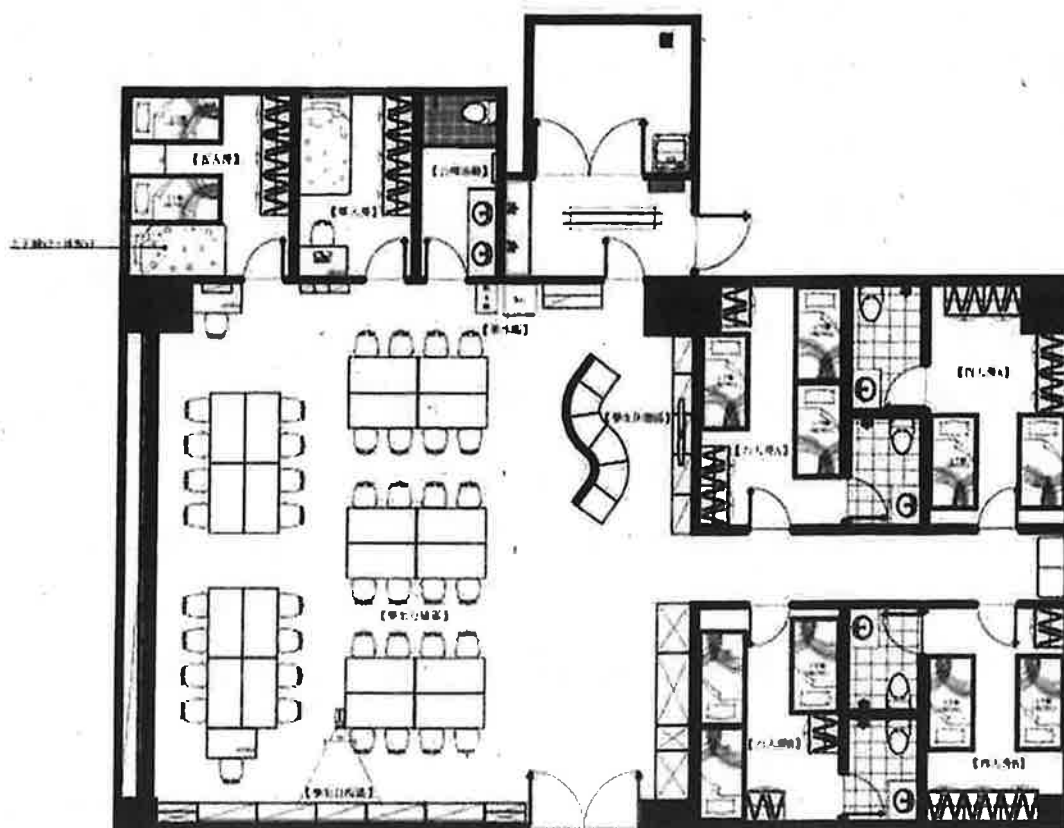
圖 1: Y802 平面圖
